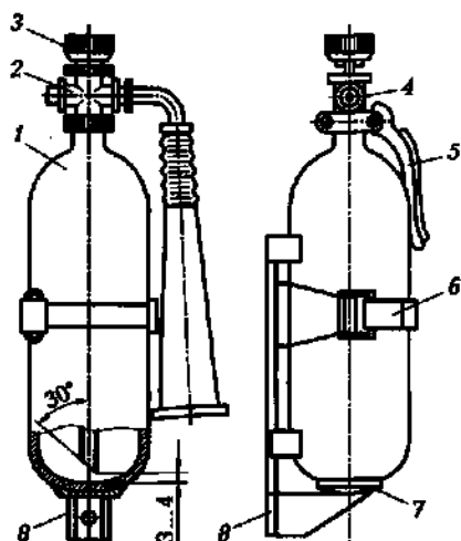
Рис. 2.3. Углекислотный огнетушитель ОУ-2:
