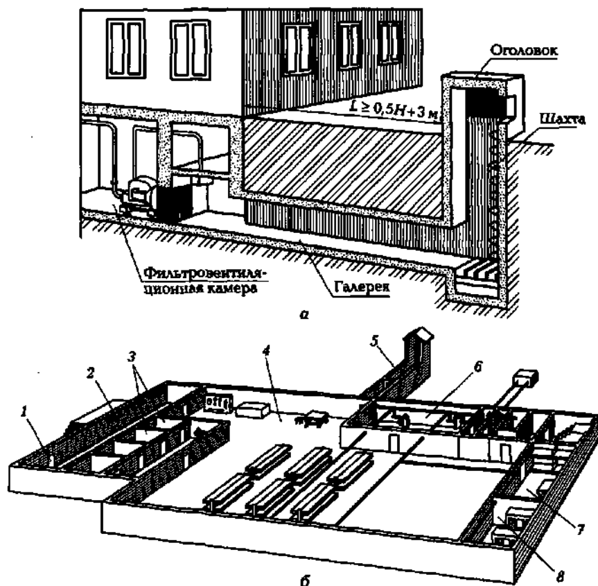
Рис. 2.9. Убежище гражданской обороны:
