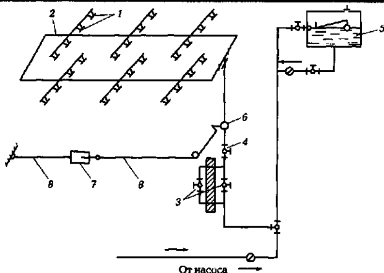
Рис. 2.7. Схема дренажной установки:
